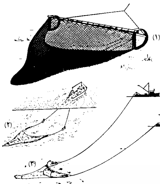
شکل ۶-۱- انواع طناب تحتانی (طناب وزنه) در تورهای ترال کفروب
